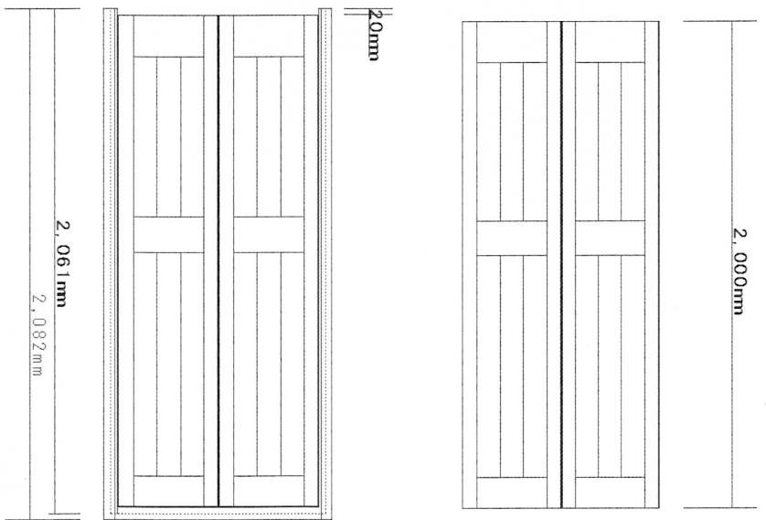
・2枚折戸断面図
